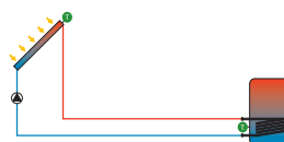
Échangeur de chaleur interne, logique de pompe
