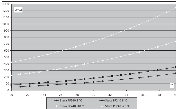
Fig. 2: Consommation d'énergie sur température ambiante pour différentes températures intérieures (PF240)
