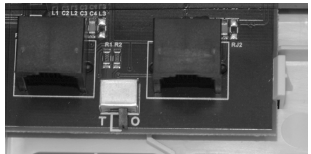
Terminaison RCC-02 désactivée (position O)
